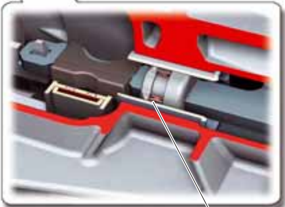
Die Abdichtung der 4 Schaltschienen erfolgt mittels doppelseitig dichtender Axialdichtelementen.
